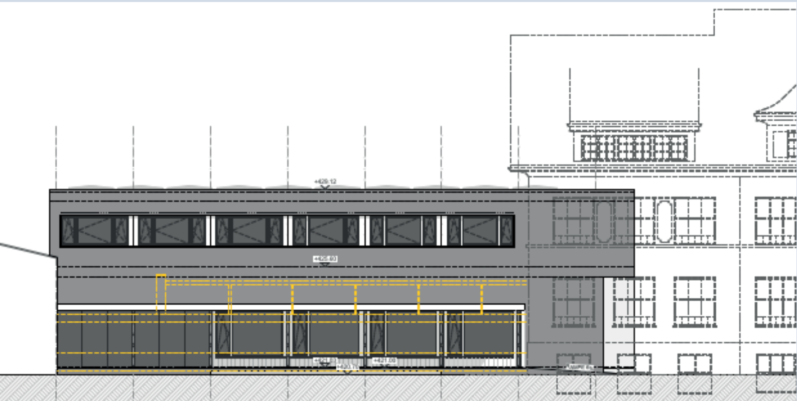
Fassaden-Schnitt Ansicht Süd
